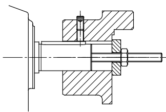
Рис. 5: Пример запрессовки
