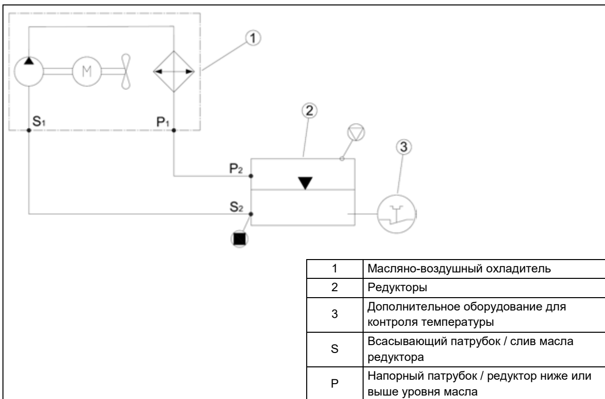
Рис. 19: Подключение охладителя
